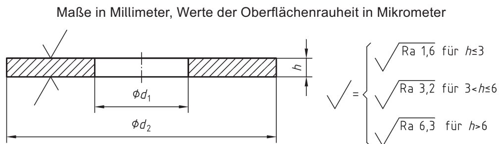
Bild 1 — Maße
